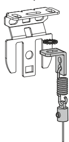
szerelősínes mennyezetre
